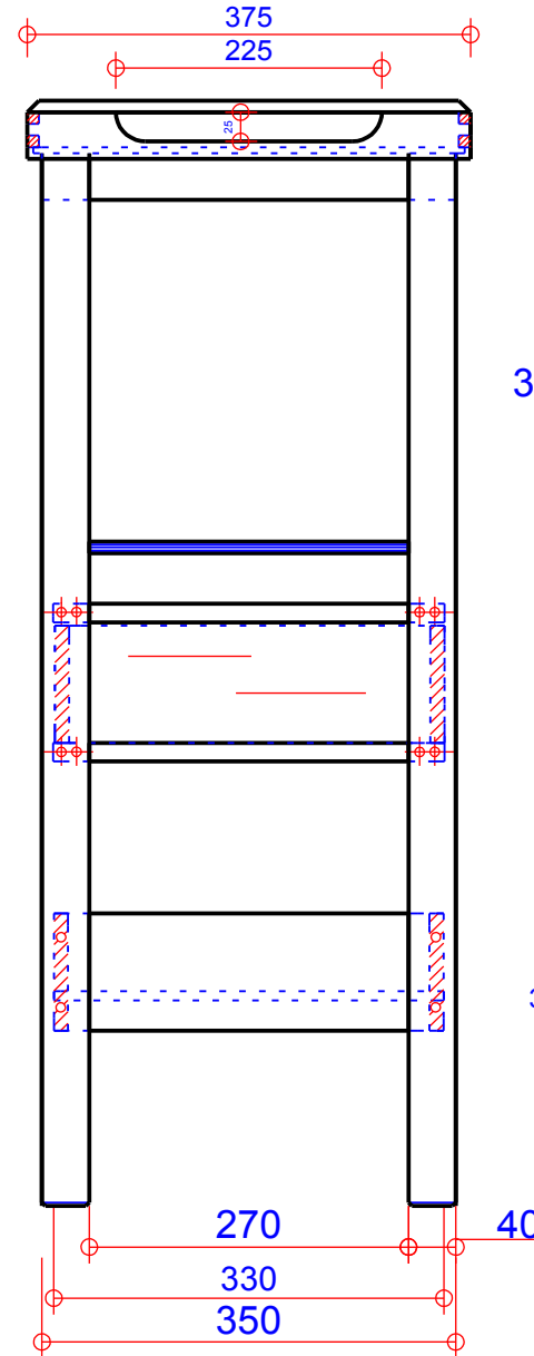
Seitenansicht
