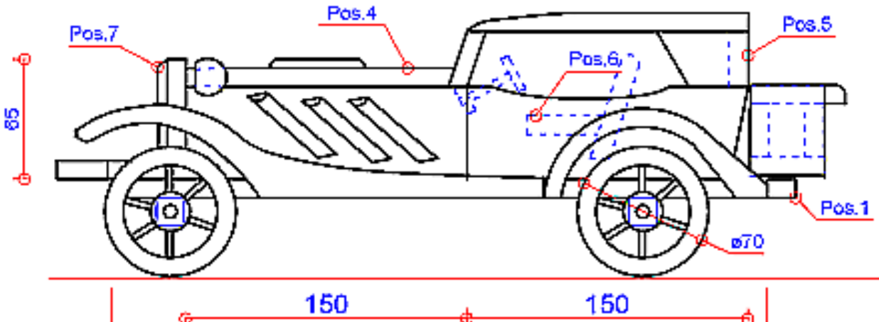
- Seitenansicht -
