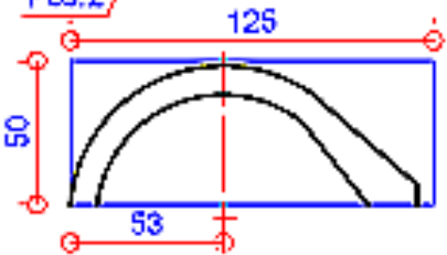
Schablone Kotflügel hinten
