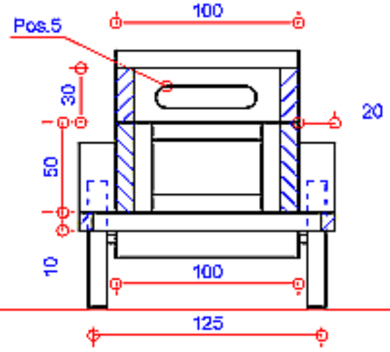
- von Vorne -
