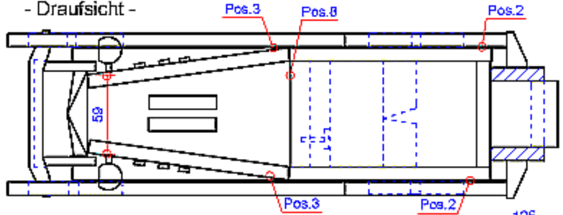
Vorderer Kotflügel
