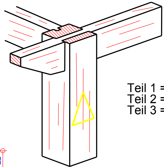
Zargenverbindung eingeschobener und gestemmter Zapfen Maßstab 1:2,5
